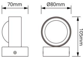
Abmessungen Leuchte
